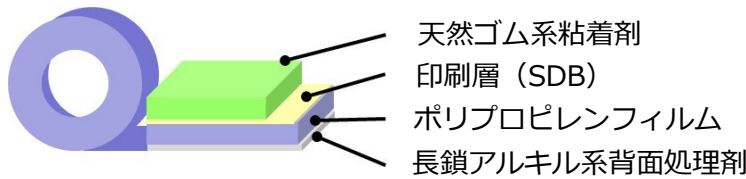
図. No.3525 テープ構成
